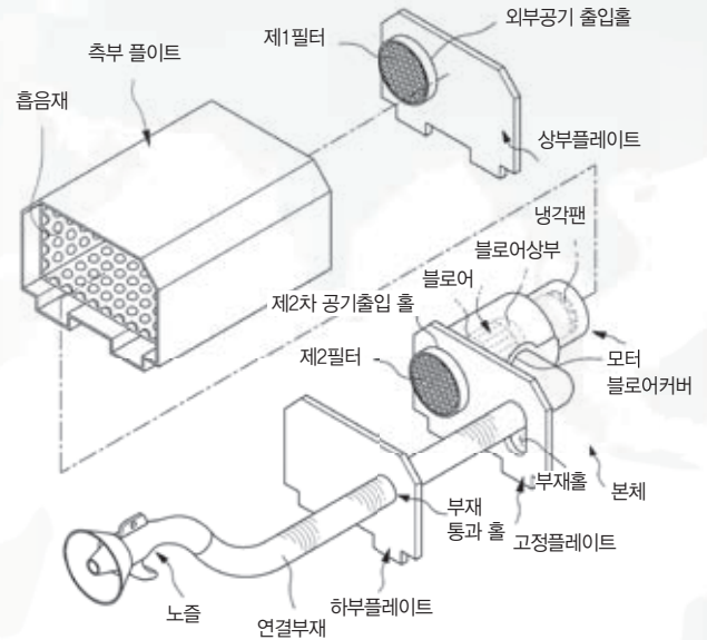
▲ 윈드건 내부명칭
