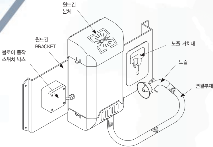
▲ 윈드건 외형도
